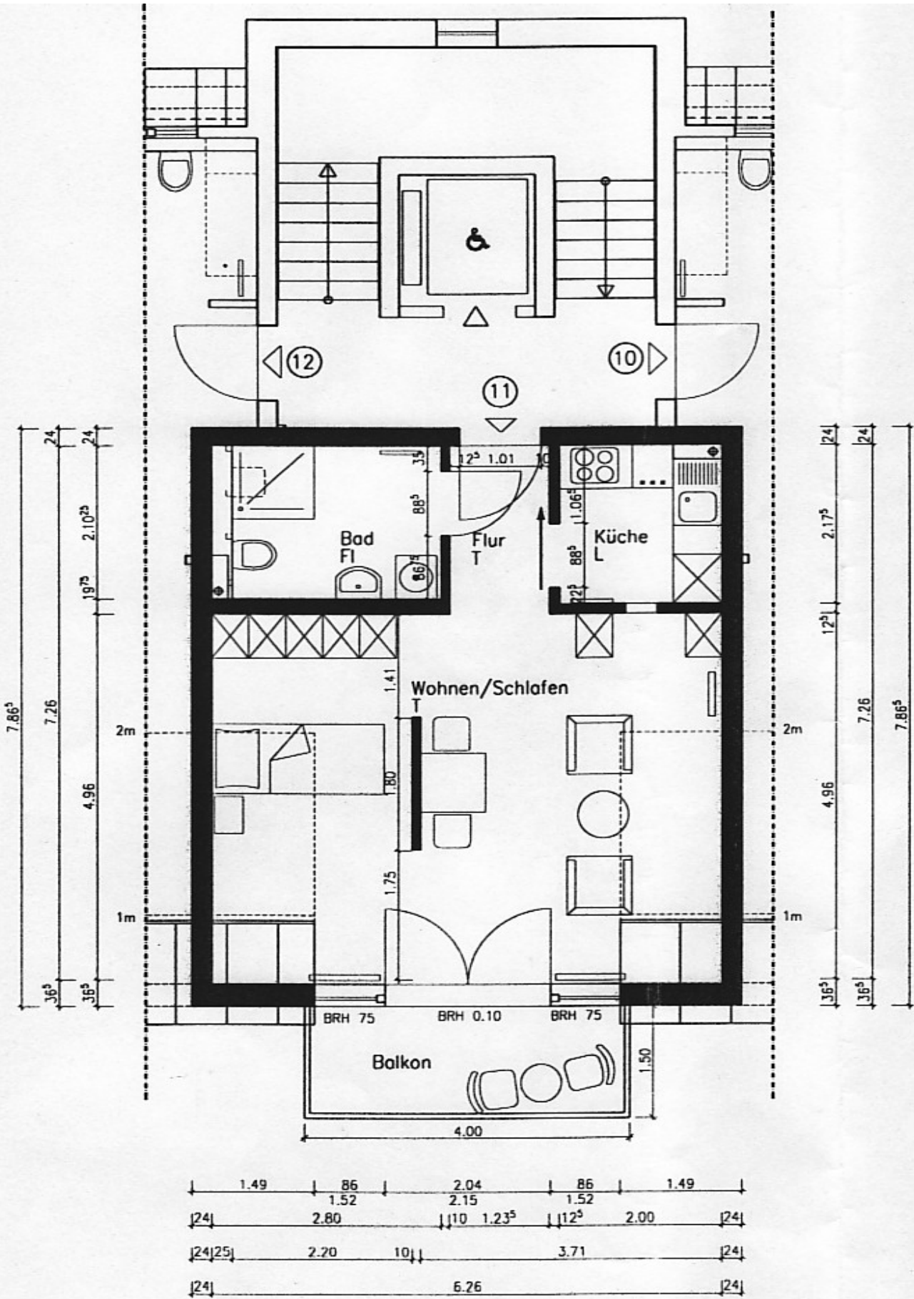
Grundriss
